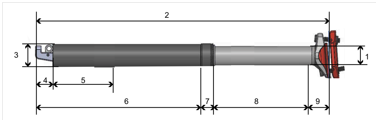
Obr. 67: Rozměrové údaje sedlovky LIMOTEC, A1L
