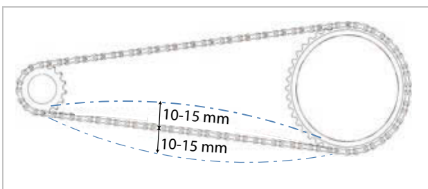
Obr. 201: Příklad kontroly napnutí řetězu: 5 mm dolů, 10 mm nahoru = výchylka 15 mm
