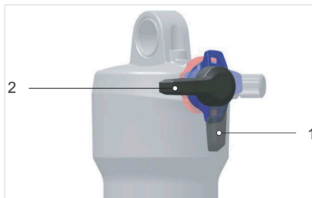
Obr. 164: Otevřená poloha (1) a prahová poloha (2) nastavovacího šroubu komprese (černá)
