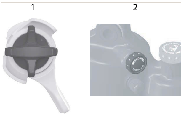
Obr. 265: Nastavovací šroub odskoku Float DPS (1) a Float X (2)
