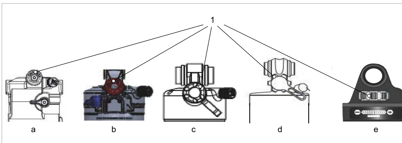
Obr. 259: Poloha nastavovacího šroubu odskoku RS Suntour (tlumič zadního odpružení) u Triair2 (a), Triair (b), EDGE-comp (c), EDGE (d) a RAISON (e)
