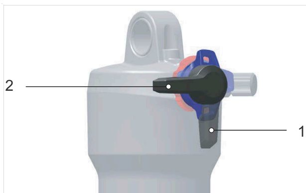
Obr. 174: Otevřená poloha (1) a prahová poloha (2) páčky
