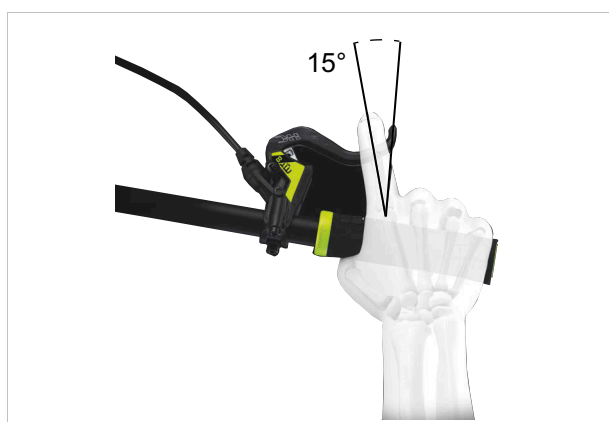
Obr. 121: Poloha ruční brzdy
