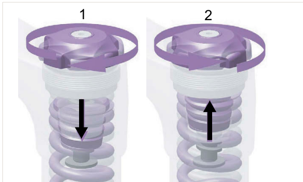
Obr. 131: Otáčení nastavovacího kolečka SAG dovnitř (1) a ven (2)
